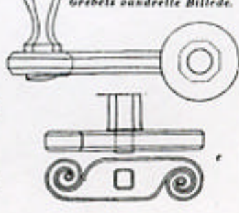
Fig. 123. Forslag til Dørgreb, Billederne a, b, c, d og e (Dørskiltene Form rettes efter Dørens Mål og Karakter).
