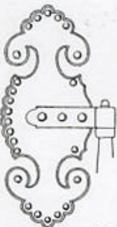
Fig. 112. Opmaaling 1:4. Dørhængsel fra Göteborg.
